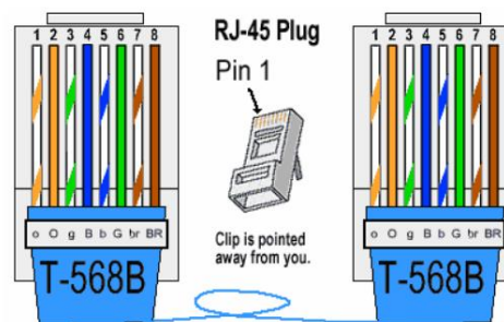
TIA/EIA 568B 接線參考圖
